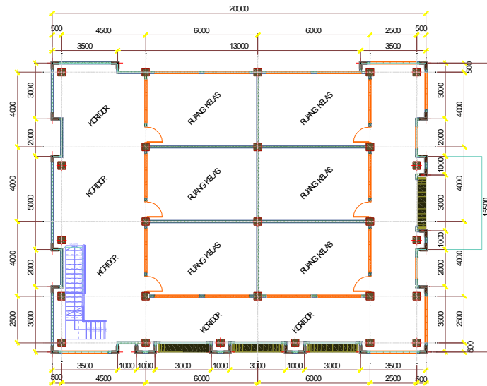
Gambar 4. Denah Lantai 2 dan 3
