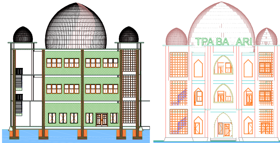
Gambar 2. Tampak Depan dan Potongan
