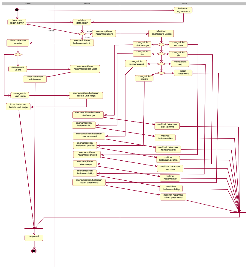
Gambar 3. Aktivitas Yang Terjadi Pada User, Admin, Dan Sistem
