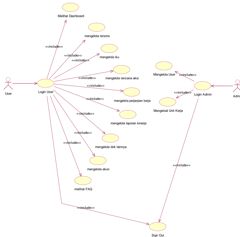
Gambar 1. Usecase Aplikasi ESAKIP
