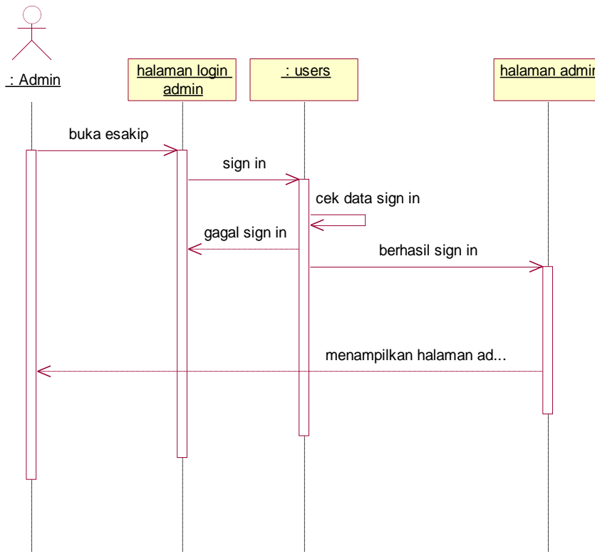
Gambar 4. Diagram Sekuen Login Admin
