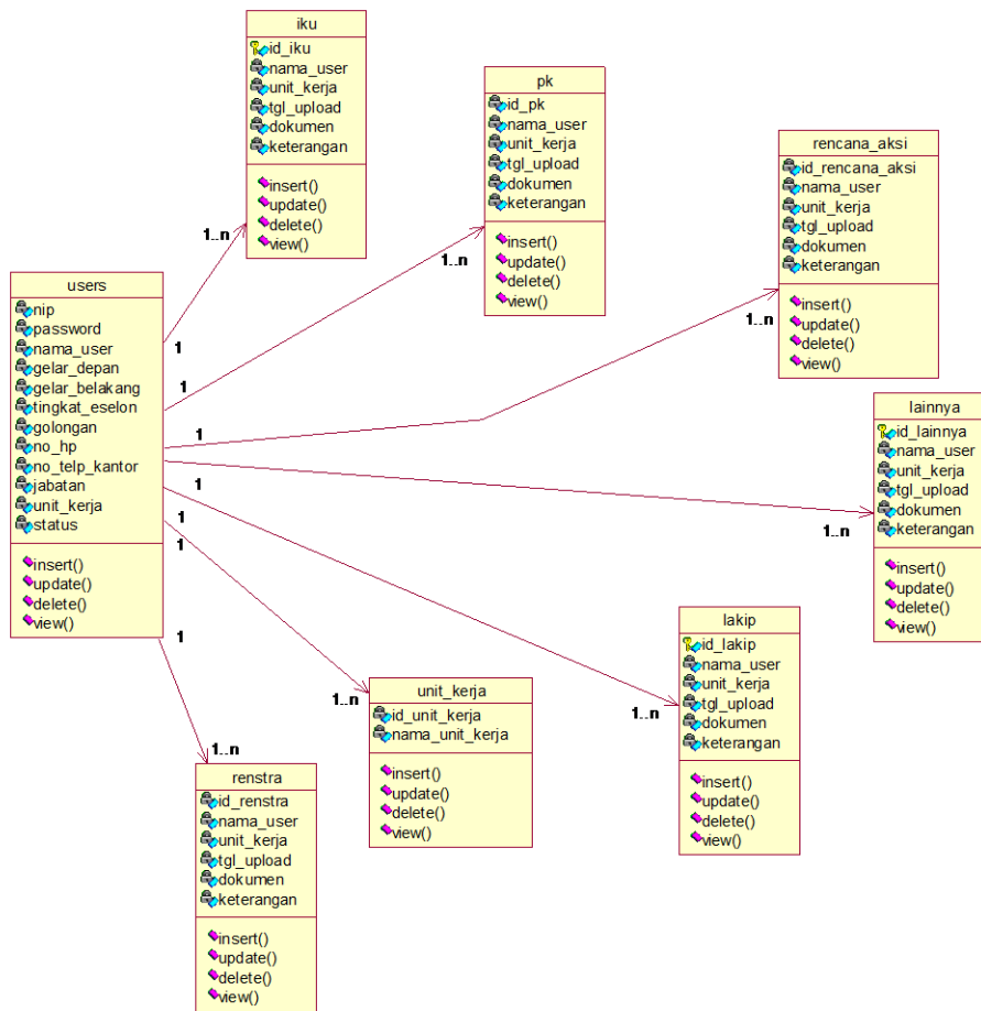
Gambar 2. Rancangan Database Aplikasi ESAKIP
